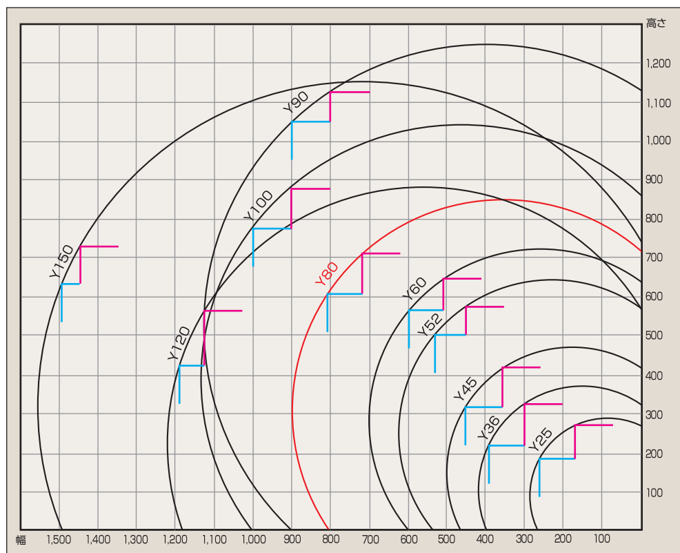
最大紐掛寸法表 単位mm
