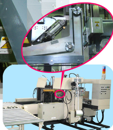
従来の上押えベルトコンベヤ
